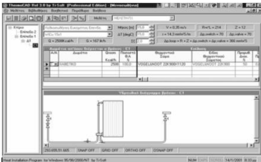
Εικόνα 8. Το λογιστικό φύλλο του προγράμματος υπολογισμού του υδραυλικού βρόχου, με τη σύνδεση τον τύπο και το μέγεθος του απαιτούμενου θερμαντικού σώματος του δωματίου
