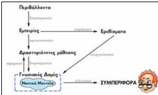
Σχήμα 1: Διαδικασία μάθησης.
