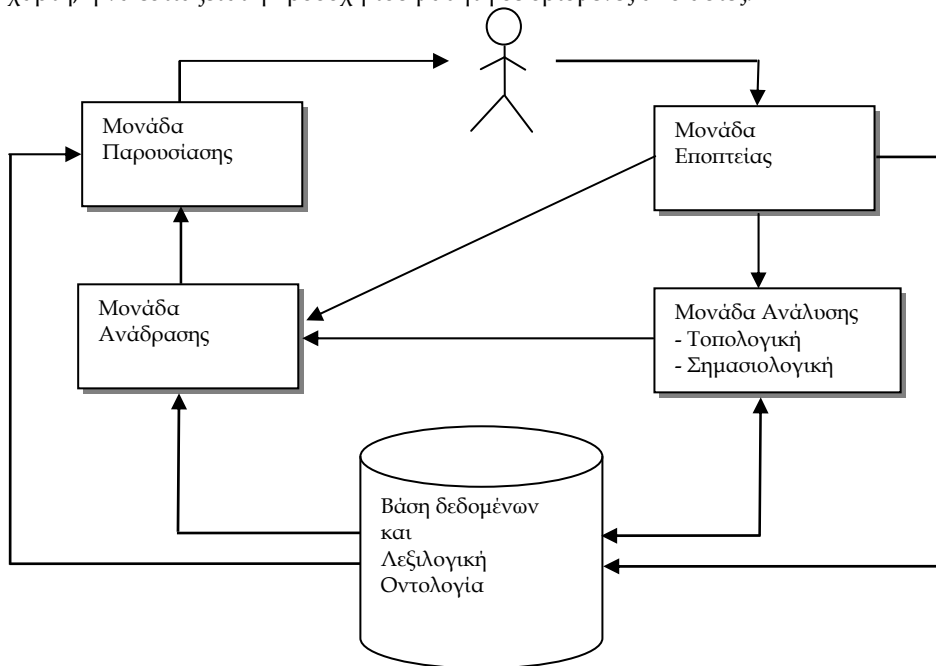
Σχήμα 2: Η αρχιτεκτονική του συστήματος
