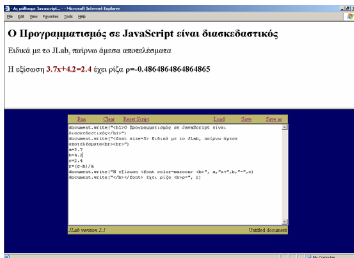
Εικόνα 1: Το περιβάλλον εργασίας «The JLab» .
