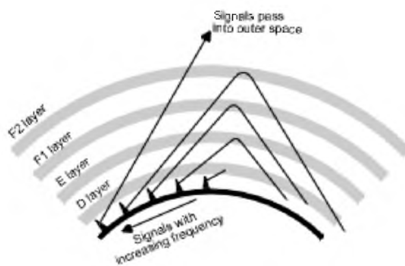
Σχήμα 13: Συμπεριφορά των στρωμάτων της ιονόσφαιρας σε σήματα με αυξανόμενη συχνότητα
