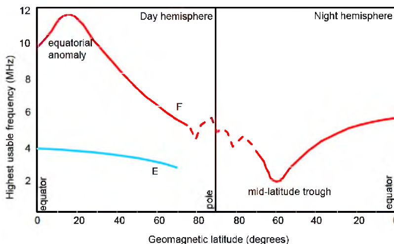
Σχήμα 16: Μεταβολές της μέγιστης ανακλώμενης συχνότητας σε σχέση με το γεωγραφικό πλάτος
