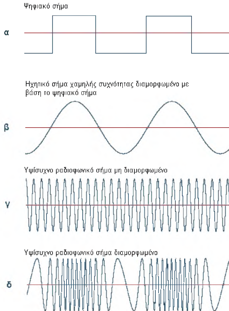
Εικόνα 4: Διαδικασία διαμόρφωσης του σήματος στο Packet Radio. Από τον υπολογιστή (α) στον πομπό (δ)
