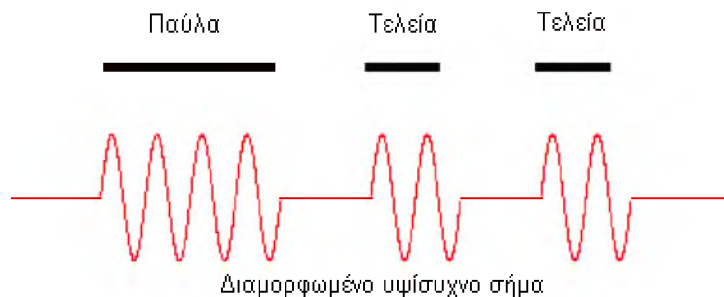
Εικόνα 5: Διαμόρφωση του σήματος στο CW
