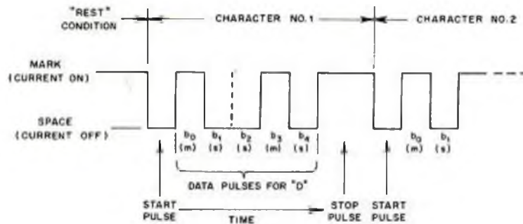
Εικόνα 7: Κωδικοποίηση του χαρακτήρα «D» στο RTTY
