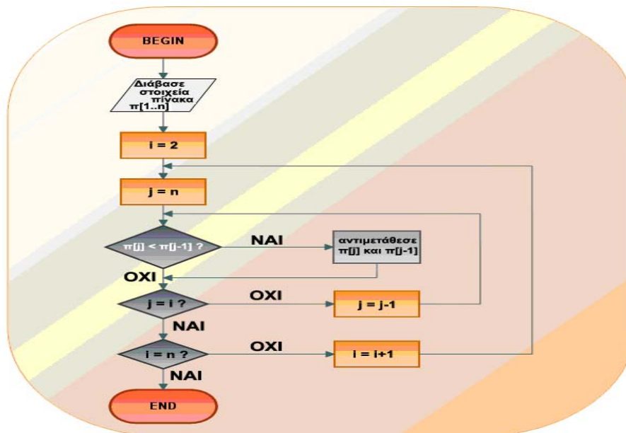
Σχήμα 3: Λογικό διάγραμμα αλγόριθμου ταξινόμησης μονοδιάστατου πίνακα σε αύξουσα σειρά με τη μέθοδο της φυσαλίδας
