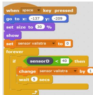
Σχήμα 2. Στιγμιότυπο κώδικα μονοδομικού επιπέδου με ατέρμονη επανάληψη
