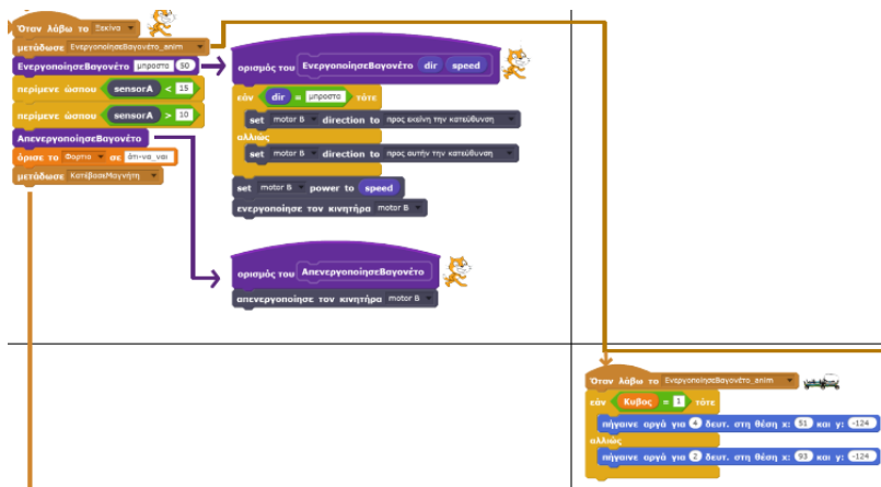
Σχήμα 4. Στιγμιότυπο κώδικα κατά το οποίο το πατρικό σενάριο συνεχίζει να εκτελείται παράλληλα με το σενάριο απόγονο
