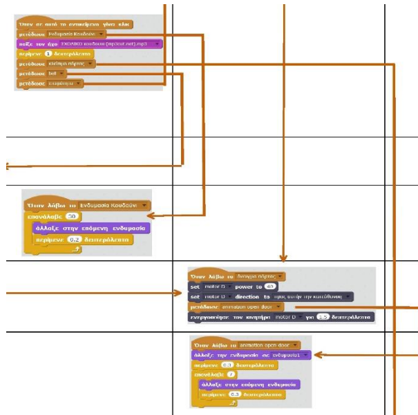
Σχήμα 3. Στιγμιότυπο κώδικα πολυδομικού επιπέδου κατά το οποίο πυροδοτούνται δύο σενάρια από διαφορετικές αιτίες
