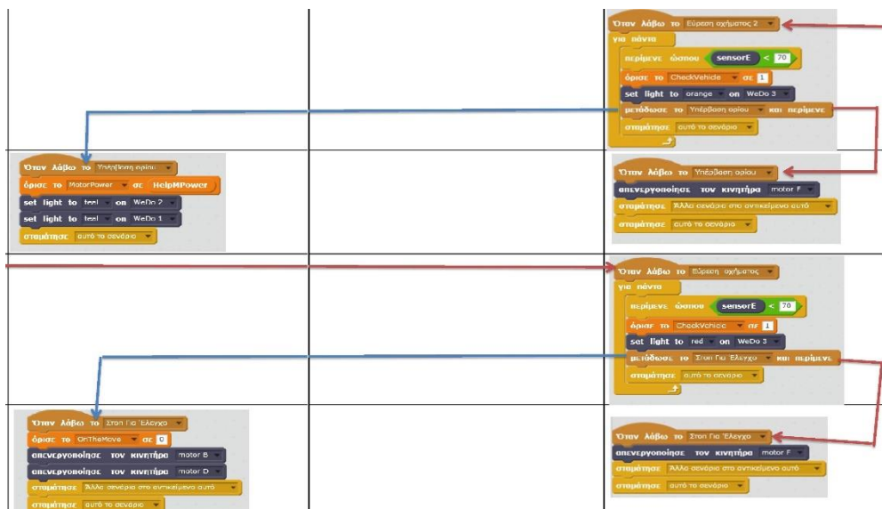
Σχήμα 8. Στιγμιότυπο ΚωδικΟράματος που επιτυγχάνεται σύγχρονη επικοινωνία με χρήση της εντολής “Μετάδωσε και Περίμενε”
