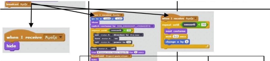
Σχήμα 1. Στιγμιότυπο κώδικα μονοδομικού επιπέδου με την πυροδότηση τριών σεναρίων από την ίδια αιτία
