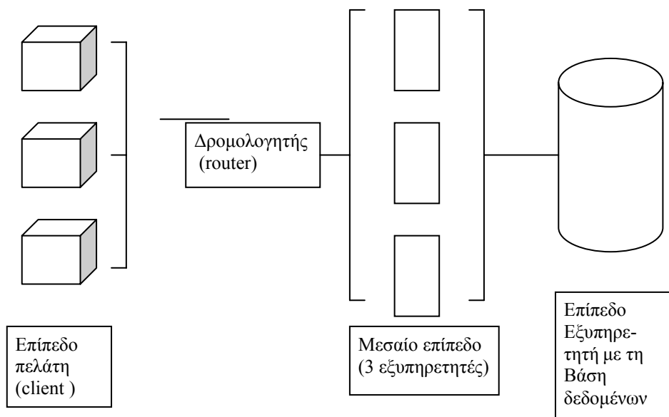
Σχήμα 3 Αρχιτεκτονική Εσωτερικού Δικτύου Διαχείρισης Μαθησιακών Αντικειμένων
