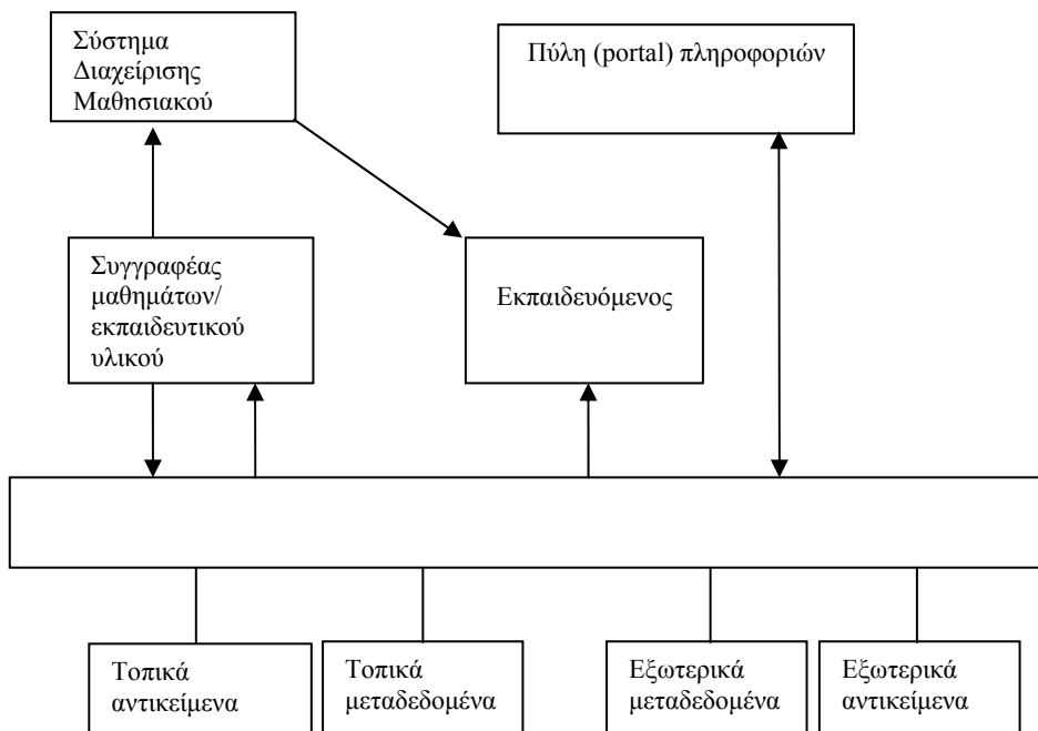
Σχήμα 2: Αρχιτεκτονική Διαχείρισης Μαθησιακών Αντικειμένων
